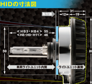
1 ライトユニットにHIDを差し込み。 2 時計回りに回してロック。 3 これで本体の取付けはOK。 4 あとは車両側のコネクターに接続で完了。
